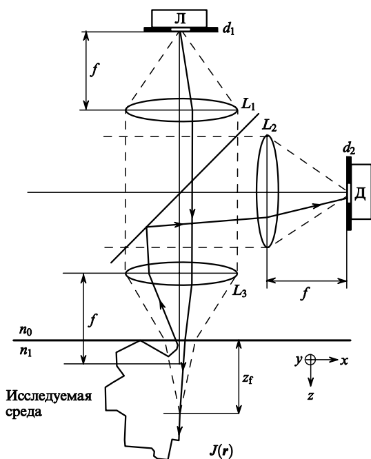
Рис.1. Схематическое представление метода конфокального зондирования: L_1, L_2, L_3 – короткофокусные линзы ( f = 8 мм), попарно образующие узкопросветный коллиматор; d_1 и d_2 – ограничивающие диафрагмы диаметром 10 мкм; z_f – глубина погружения в среду точки фокуса; Л – лазерный источник; Д – приемник оптического излучения; n_0 и n_1 – коэффициенты преломления внешней и исследуемой сред.
