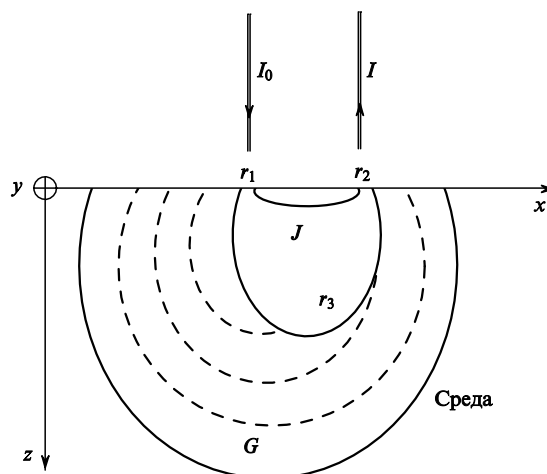
Рис.2. Схема области пространственного распределения падающего излучения G в случайно-неоднородной многослойной сильно рассеивающей свет среде при волоконно-оптическом зондировании последней: J (J \subset G) – область пространственного распределения эффективных оптических путей фотонов, характеризующая область локализации детектируемого сигнала; r_1 – координата входа пакета фотонов в среду; r_2 – координата выхода пакета фотонов из среды; r_3 – координата исследуемой среды.
